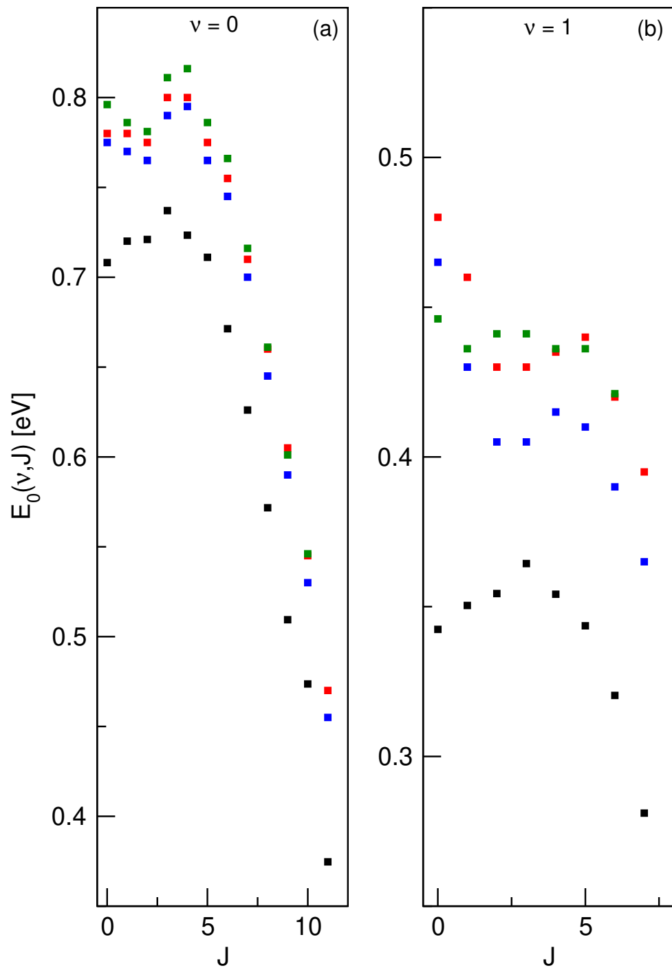
\text{H}_2 + \text{Cu}(111)
