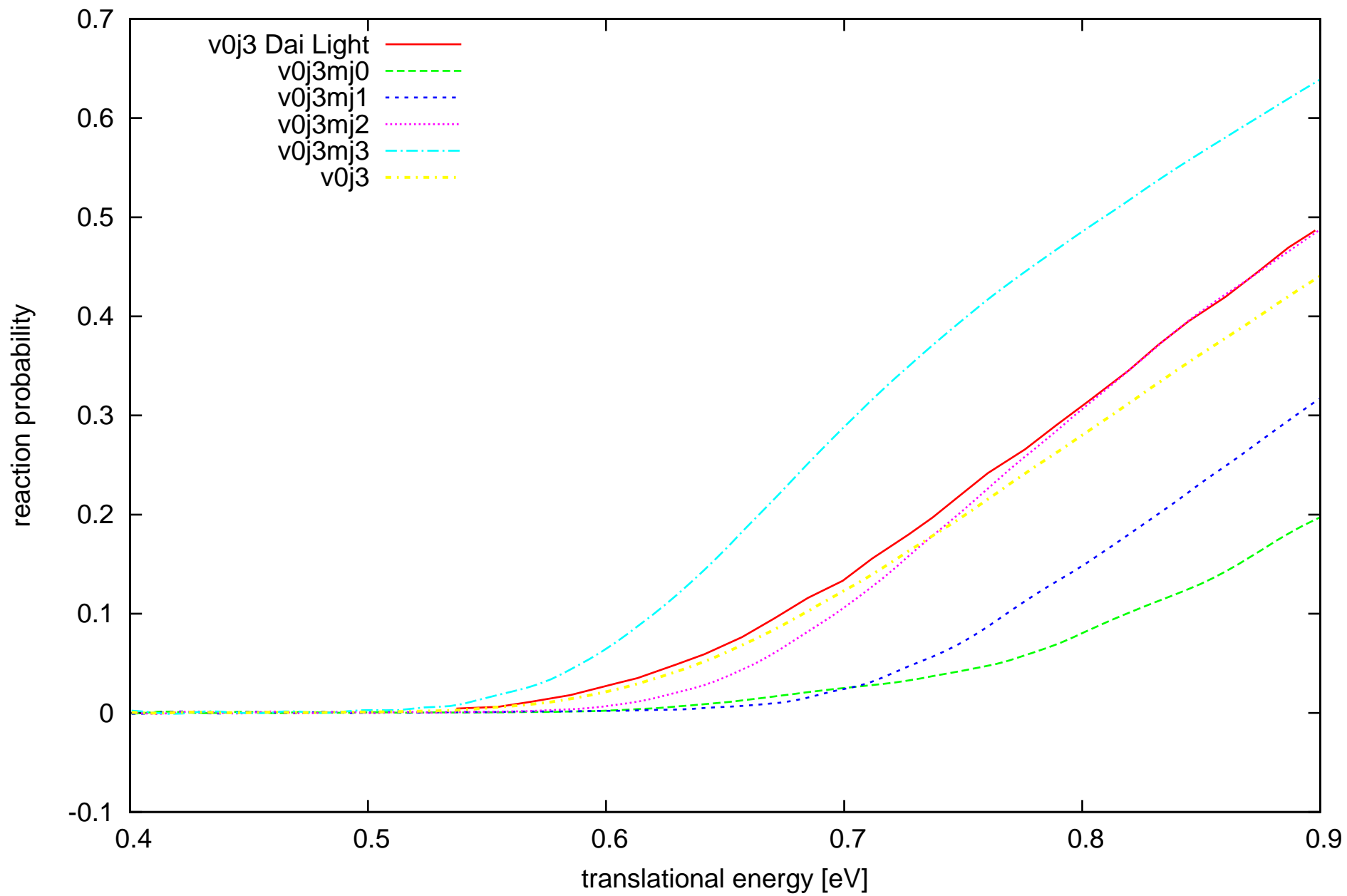
6D QD Dai Zhang LEPS PES v0j3
