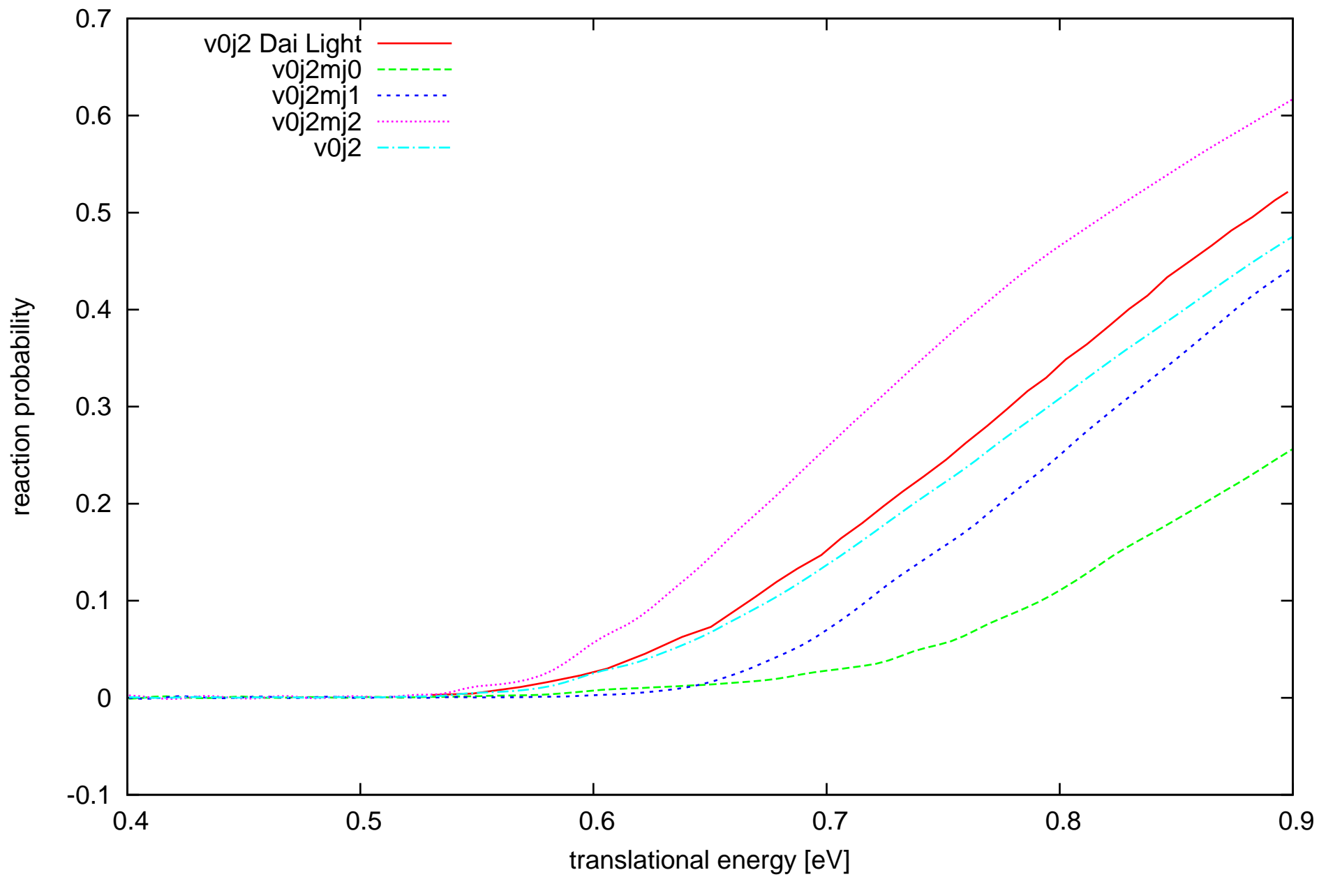
6D QD Dai Zhang LEPS PES v0j2
