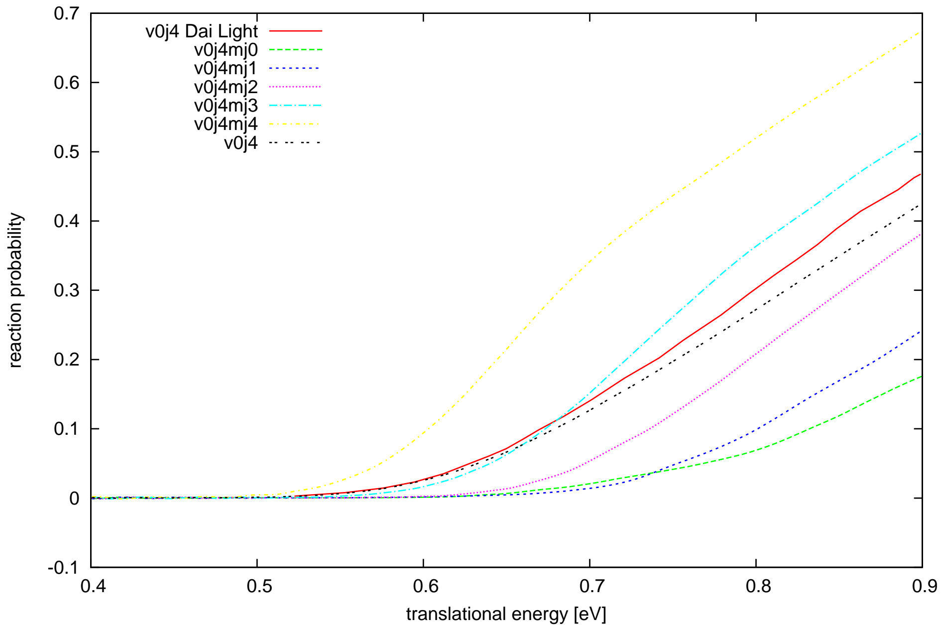
6D QD Dai Zhang LEPS PES v0j4
