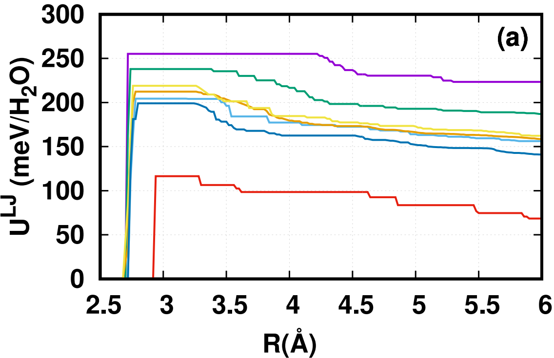
TIP4P/2005
